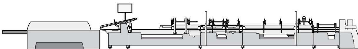
Sammel und Presseinrichtung Überleitstation Faltstation Kombifaltmodul Vorbrechstation Ausrichtmodul Einleger
